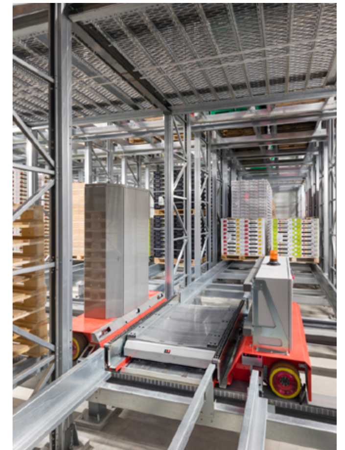
AUTOMATISIERTES LAGERSYSTEM MIT MOTHER-CHILD SHUTTLE-LÖSUNG AUTOMATED STORAGE SYSTEM WITH MOTHER-CHILD SHUTTLE SYSTEM
